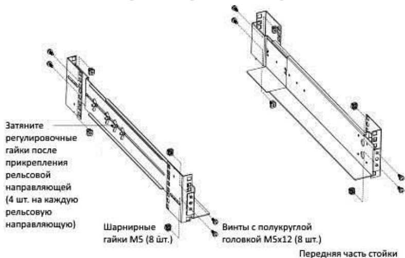
Рис. 2 Закрепление направляющих
